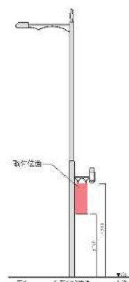
■街路灯取付図
